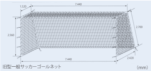
旧型一般サッカーゴールネット (mm)
