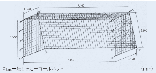
新型一般サッカーゴールネット (mm)
